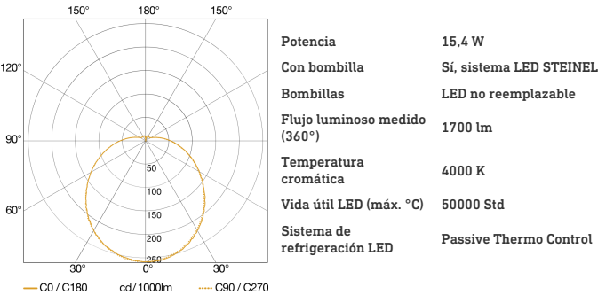
Curva de dispersión lumínica
