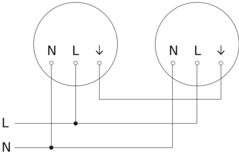
Diagrama electrónico interconexión maestro-maestro
