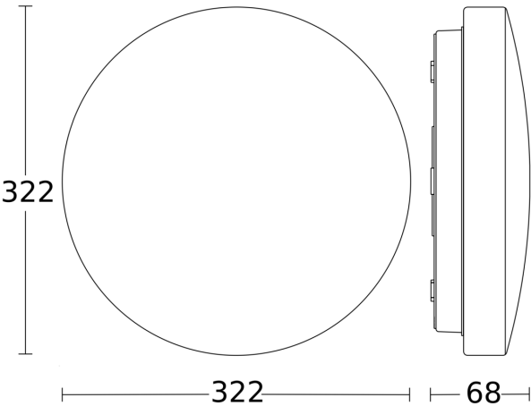
Dibujo acotado
